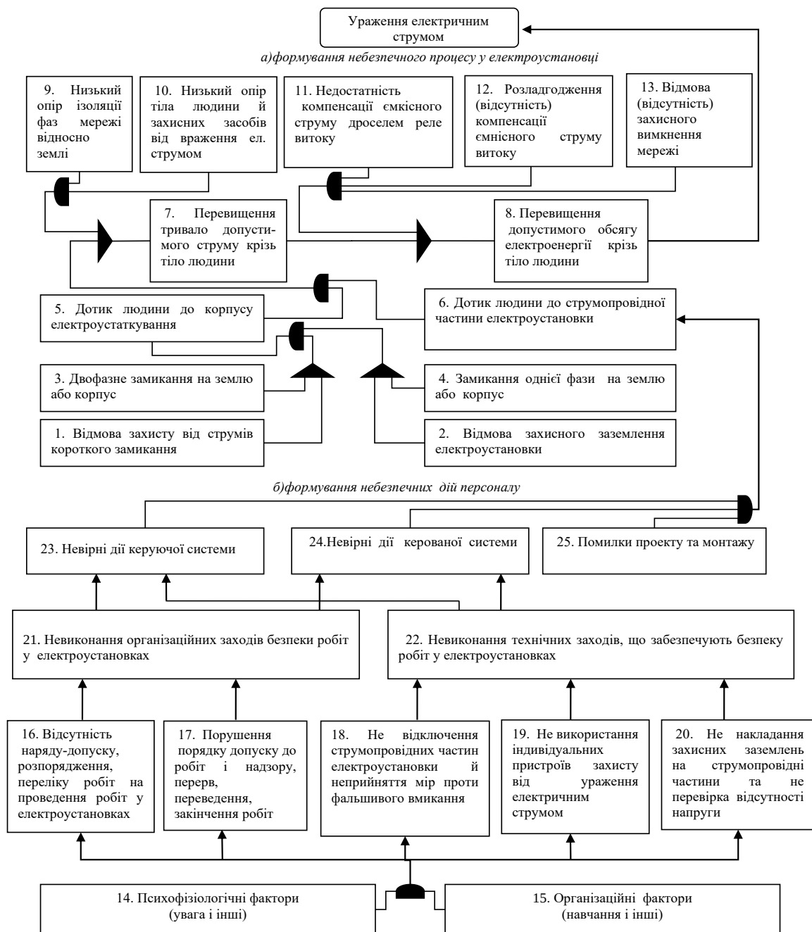
Рис. 3. Логічна модель реалізації небезпеки ураження електричним струмом у системі «людина –залізорудне виробництво – електротехнічні комплекси»
