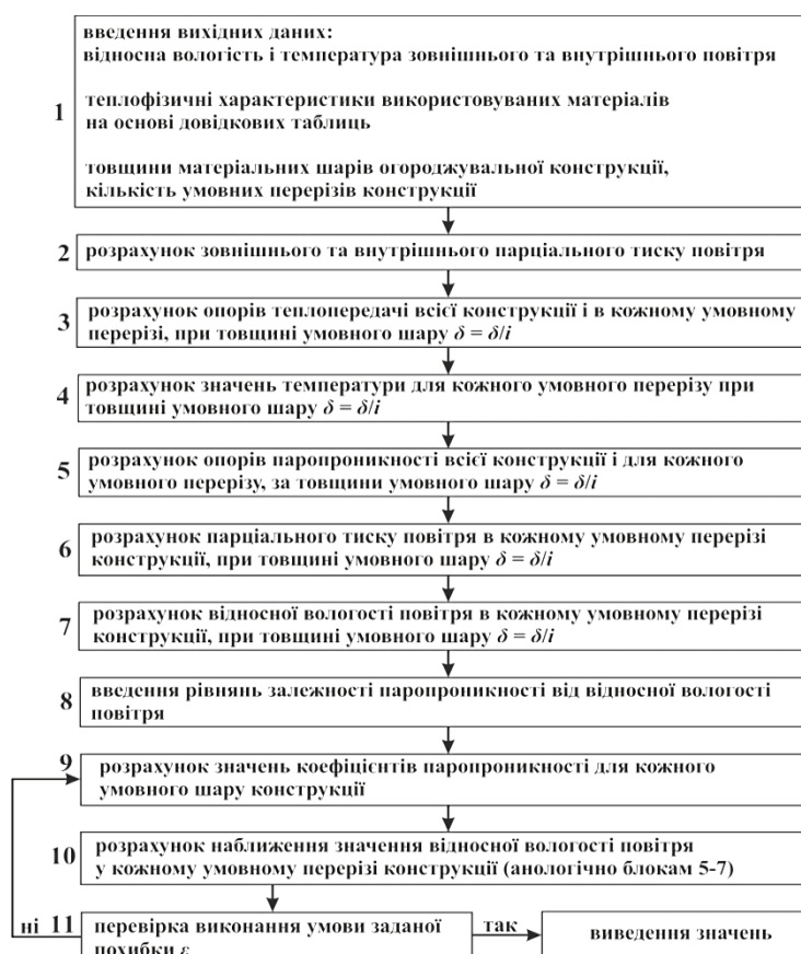
Рис. 3. Алгоритм методу розрахунку паропроникності матеріальних шарів конструкції
