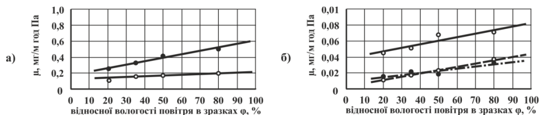
Рис. 2. Залежність коефіцієнту паропроникності \mu (мг/м-год·Па) матеріала від середньої відносної вологості повітря у зразку \varphi_{сер} %
