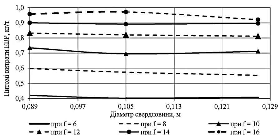
Рис. 3. Залежності питомих витрат вибухової речовини на відбійку від діаметру свердловини та коефіцієнту міцності руди (за удосконаленою методикою)
