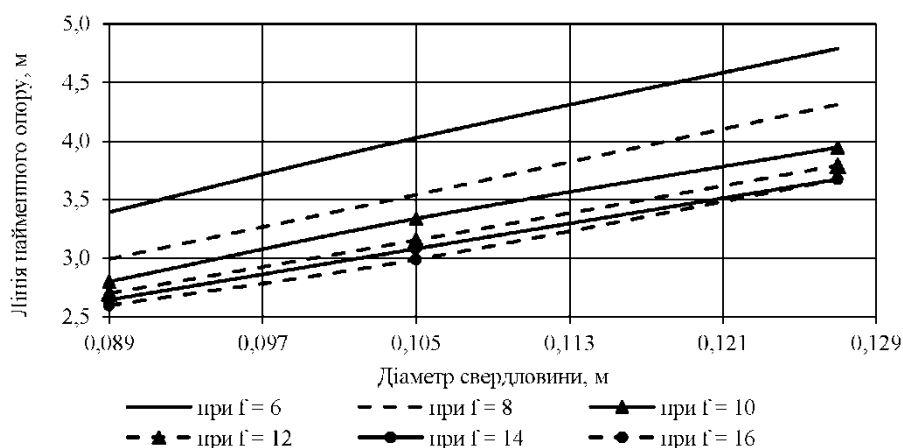
Рис. 2. Залежності лінійного найменшого опору від діаметру свердловини та коефіцієнту міцності руди (за удосконаленою методикою)
