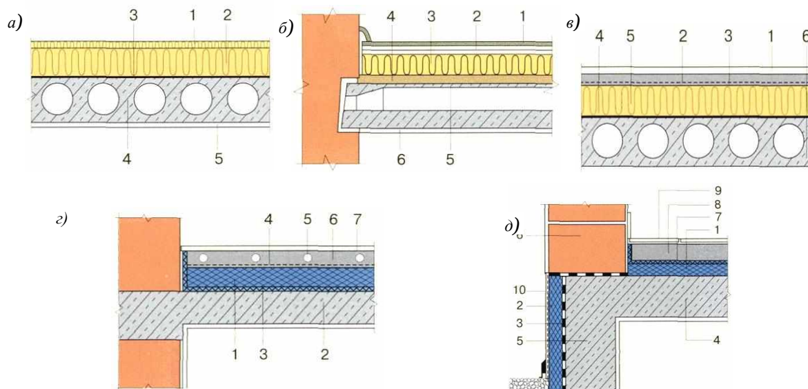
Рис. 2. Конструкції вузлів по перекриттю: а – горищне перекриття (1 – скловатна плита RKL – 30 мм; 2 – скловатна плита KL – 125 мм; 3 – поліетиленова плівка; 4 – залізобетонна плита; 5 – штукатурка); б – міжповерхове перекриття з безшовною підлогою (1 – покриття підлоги; 2 – дерев'яно-стружкова плита – 2 шари; 3 – скловатна жорстка плита – FLO – 40 мм; 4 – піщана засипка із зв'язкою; 5 – залізобетонна пустотна плита; 6 – вапняно-цементна штукатурка); в – перекриття над проїздом (1 – покриття підлоги; 2 – стягування; 3 – арматурна сітка; 4 – поліетиленова плівка; 5 – скловатні плити OL-YK, OL-K – 150 мм; 6 – залізобетонна плита); г – міжповерхове перекриття з обігрівом підлоги (1 – екструдований пінополістирол Floomate; 2 – залізобетонна плита; 3 – екструдований пінополістирол Styrofoam; 4 – поліетиленова плівка; 5 – ogrівальні труби; 6 – стягування; 7 – покриття підлоги); д – перекриття над холодним підвалом (1 – екструдований пінополістирол Floomate; 2 – екструдований пінополістирол Styrofoam; 3 – гідроізоляція; 4 – залізобетонна плита; 5 – стіна підвального приміщення; 6 – стіна зовнішня; 7 – екструдований пінополістирол Styrofoam; 8 – стягування; 9 – покриття підлоги; 10 – обробка цоколя)
